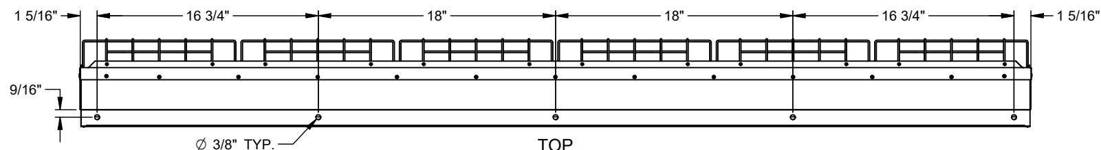
TOP 1:10
