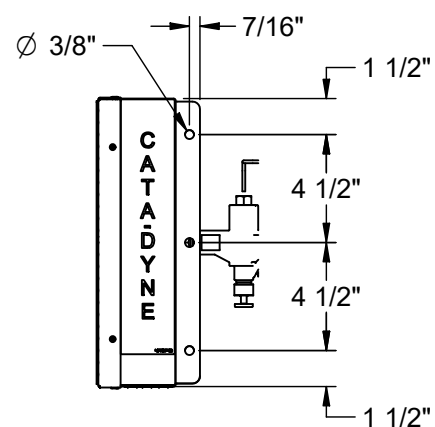
SIDE 1:8
