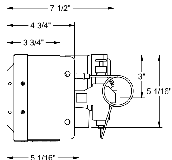
RIGHT SIDE 1:4
