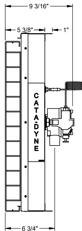
SIDE 1:8
