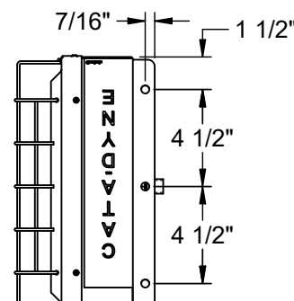
SIDE 1:8
