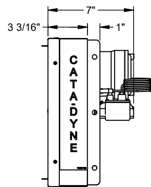
SIDE 1:8
