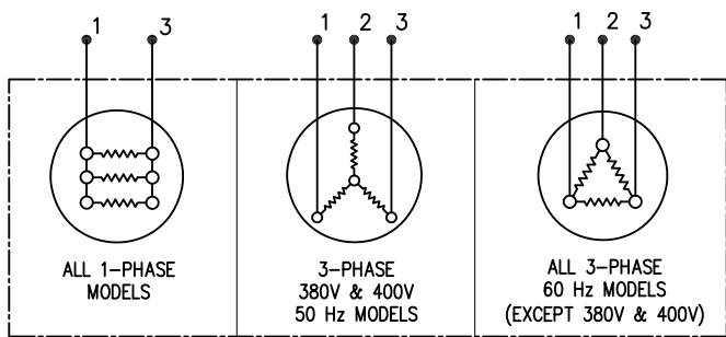
ELEMENT WIRING
