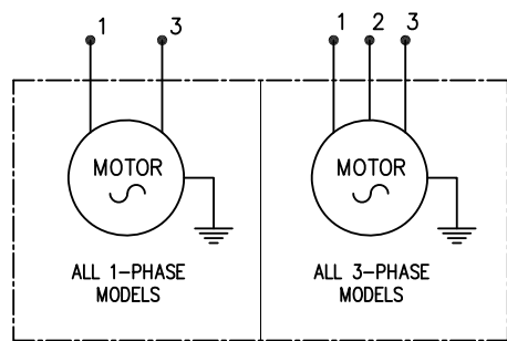
MOTOR WIRING
